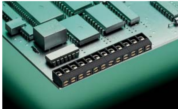
AK(Z) 500/.. DS - 5,0 (5,08) - H - grey
